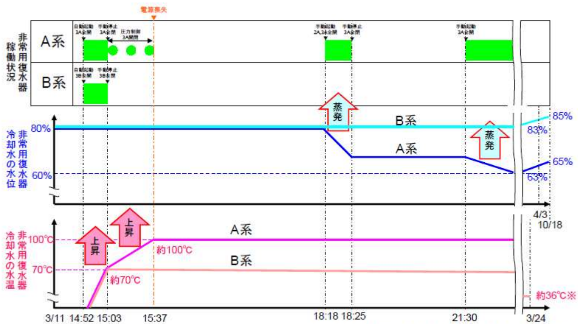
図3 ICの冷却水水位、水温と稼働状況の関係(イメージ)
